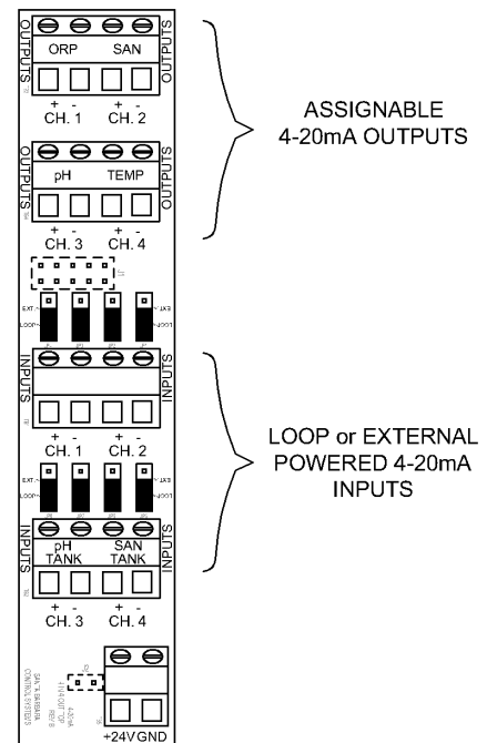
OPTIONAL 4 IN 4 OUT 4-20mA MODULE
