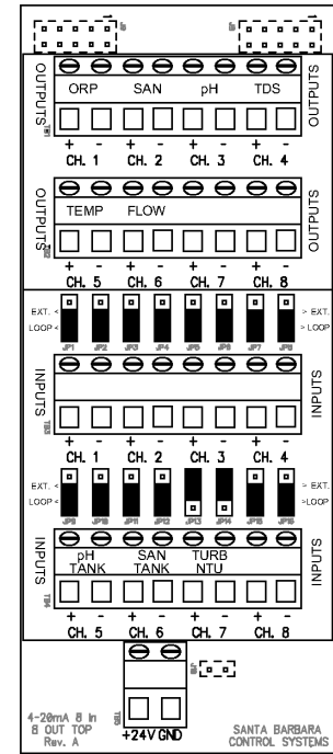
OPTIONAL 8 IN 8 OUT 4-20mA MODULE
